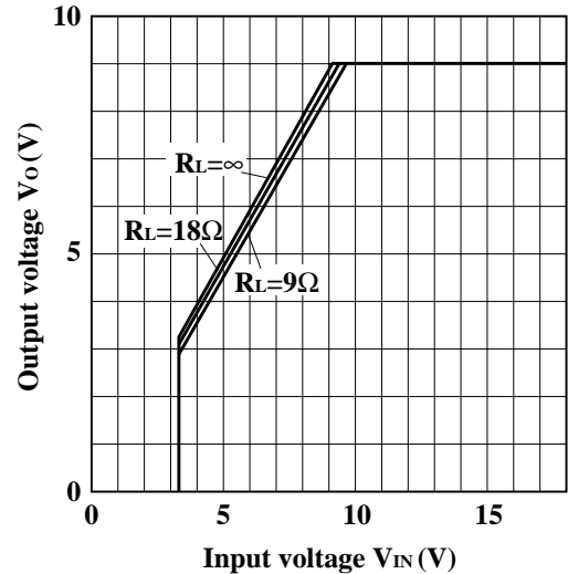
Fig.12 Output Voltage vs. Input Voltage (PQ09RF1/PQ09RF11/PQ09RF1V)
