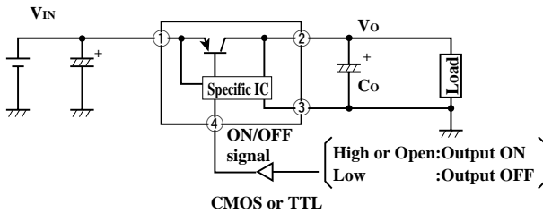
PQ05RF1/PQ05RF11 Series
